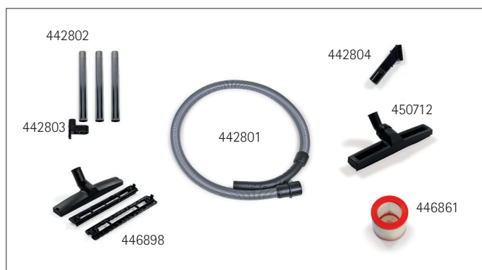
KIT D'ACCESSOIRES Ø32 (EN SÉRIE)
